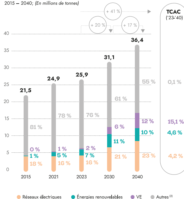
Perspectives de la demande de cuivre raffiné (1) par secteur dans le scénario d'engagement annoncé par l'AIE 2015 – 2040; (En millions de tonnes)
